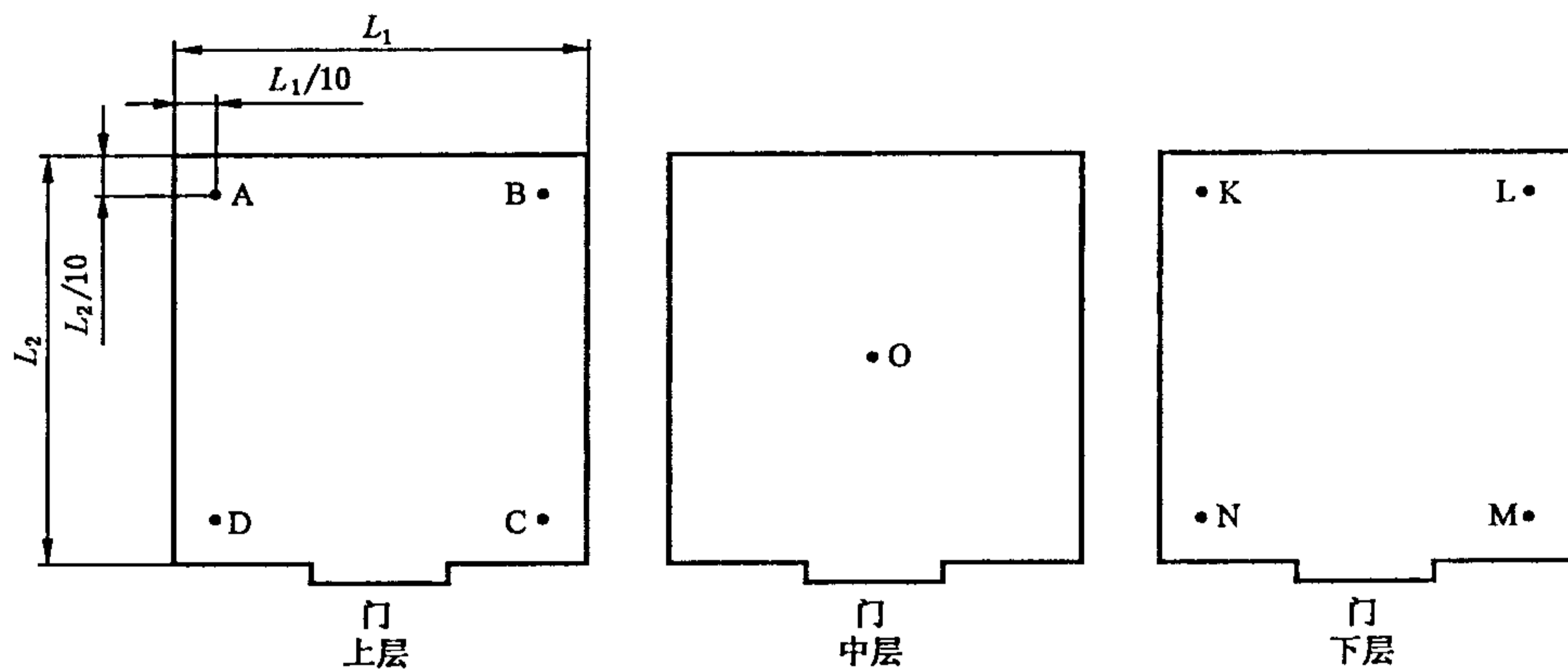
A,B,...,M,N——温度测试点
